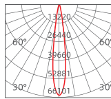
配光参数： IES
